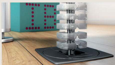
Исполнение Unit с гибким кабель-каналом для монтажа в пол. Detail of ground Unit and Vertebra.
